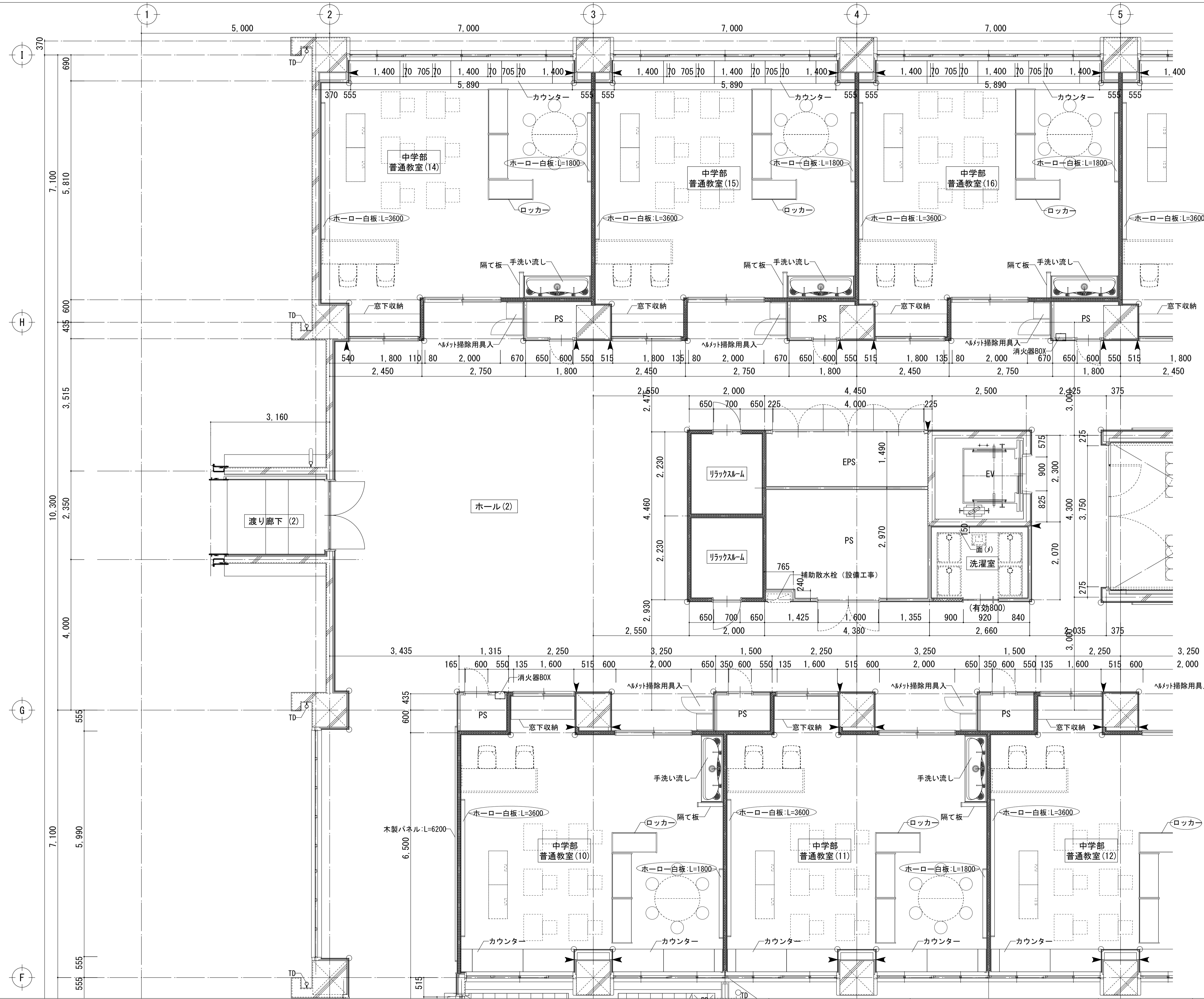
3階平面詳細図(5) S=1/50
